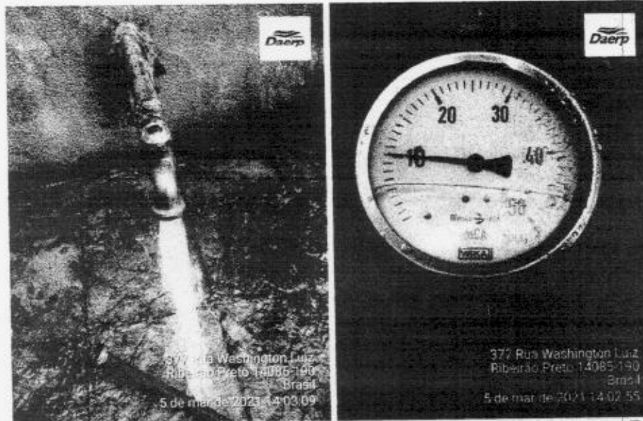
Figura 1 – Verificação das condições de fornecimento de água na Rua Washington Luiz, nº 377, e aferição de pressão (10 mca) no dia 05/03/2021.
