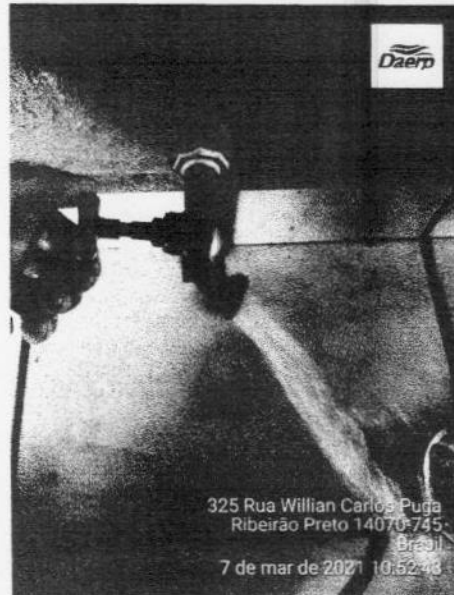
Figura 1 – Verificação das condições de fornecimento de água na Rua Willian Carlos Puga, n° 325, e aferição de pressão (17 mca) no dia 07/03/2021.
