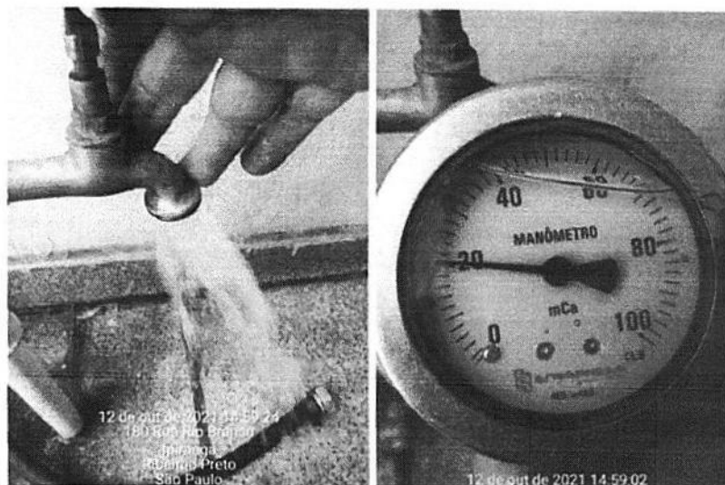
Figura 1 – Visita técnica na Travessa Barras, nº 537, Bairro Ipiranga, para verificação das condições do abastecimento de água e aferição de pressão (20 mca), no dia 12/10/2021.
